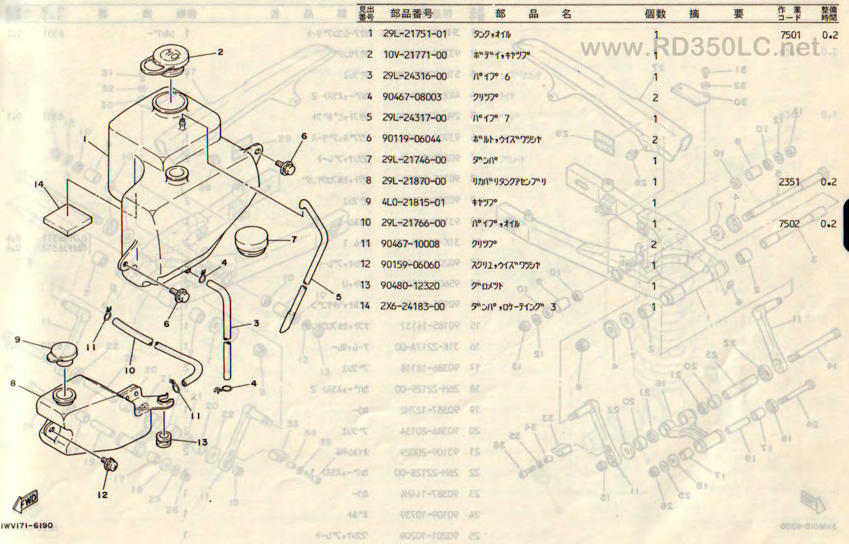
FIG. 19 オイルタンク
